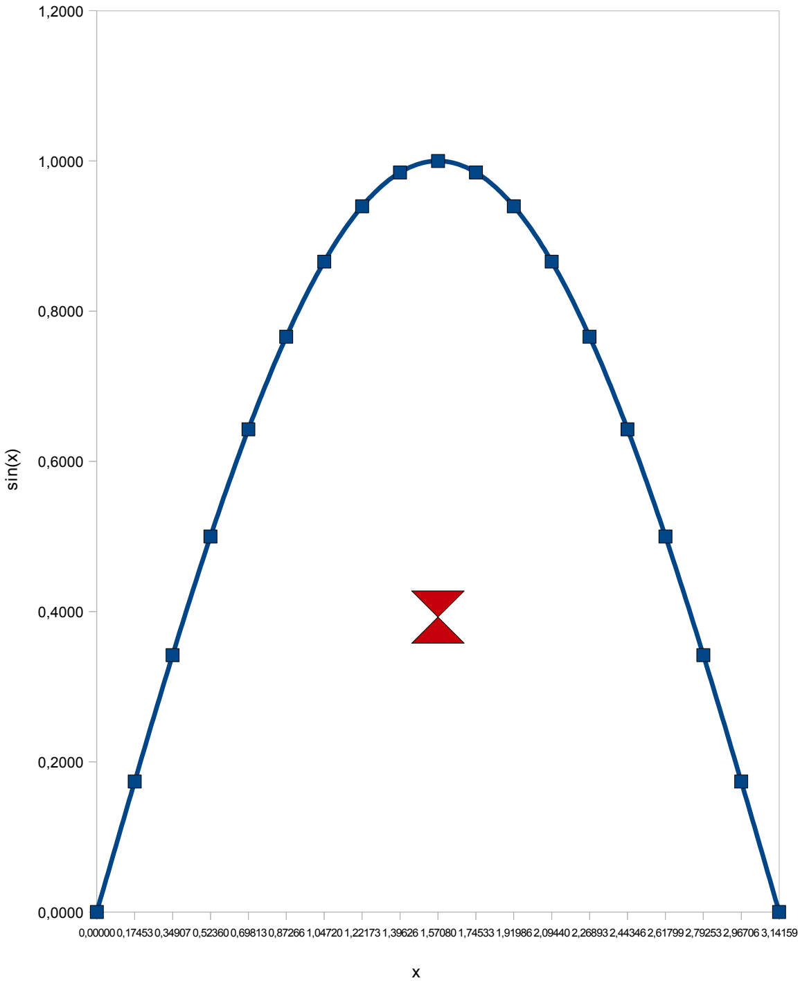
Flächenschwerpunkt \sin(x)
